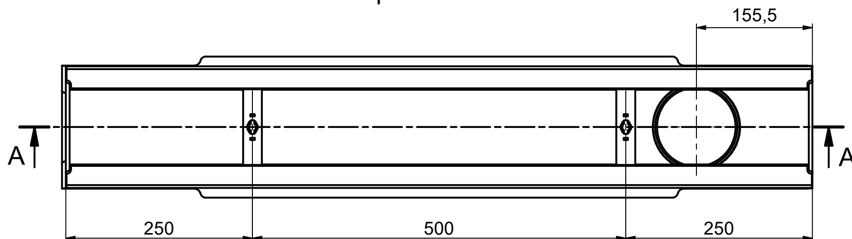
Draufsicht / top view / vue de dessus
