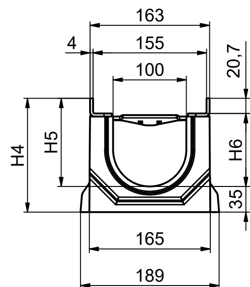
Ansicht Feder / view tongue / vue languette
