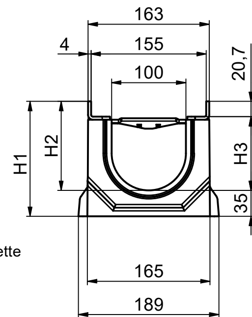
Ansicht Nut / view groove / vue rainure
