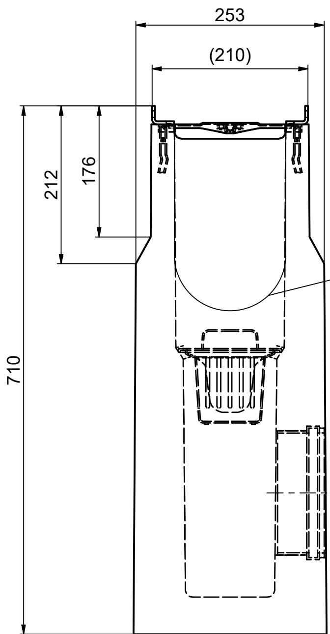
Seitenansicht / side view / vue de côté
