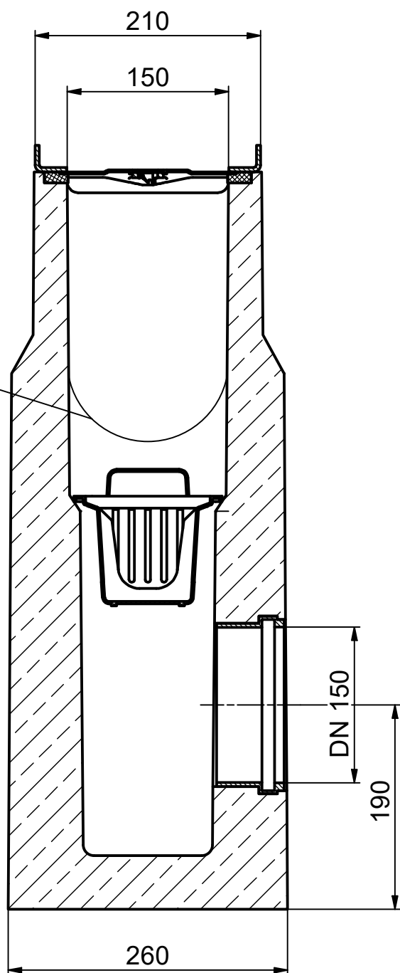
Schnitt / section / coupe B-B
