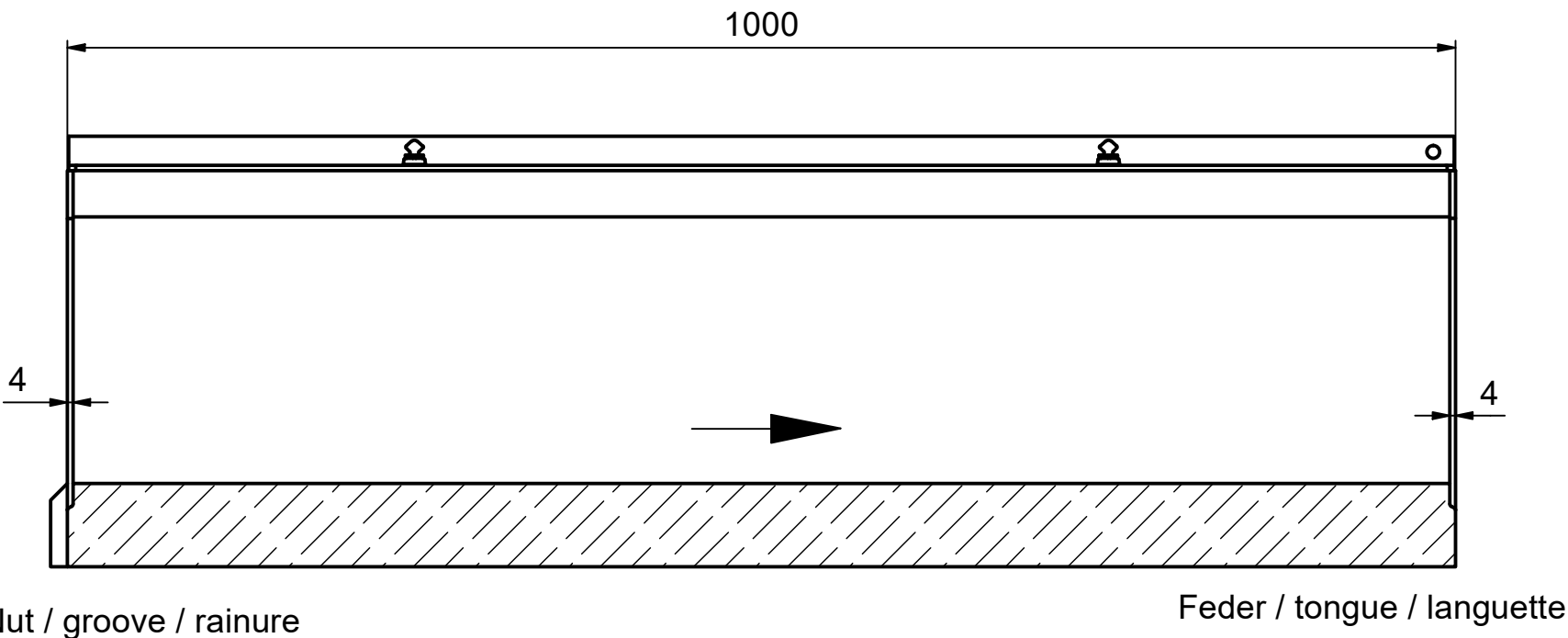
Schnitt / section / coupe A-A
