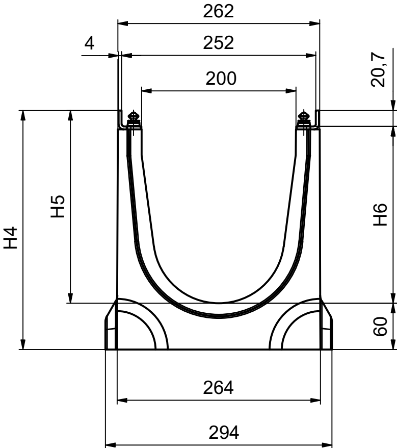
Ansicht Feder / view tongue / vue languette
