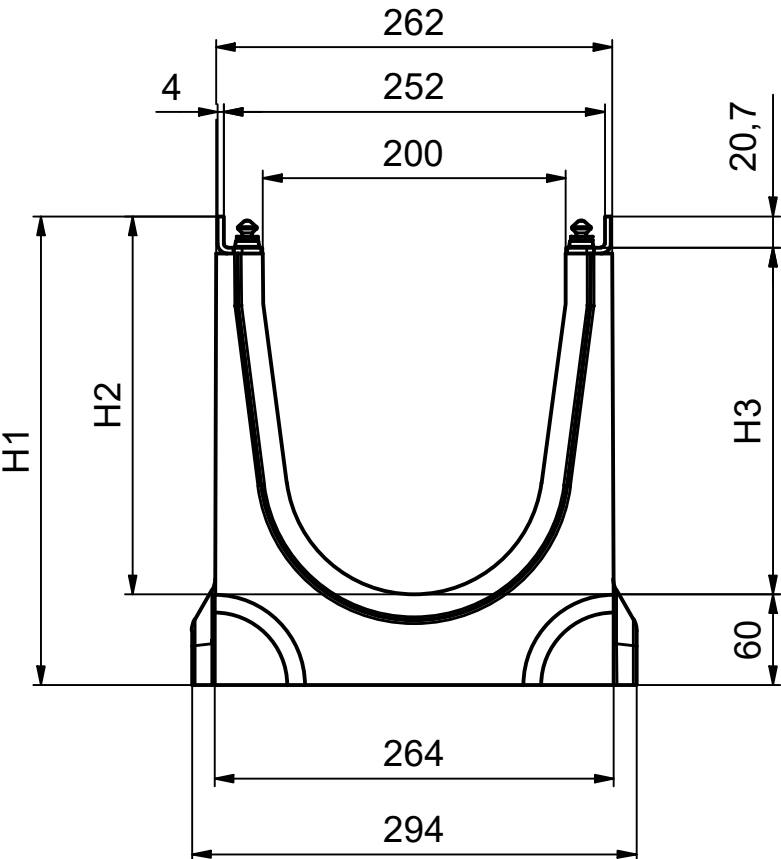
Ansicht Nut / view groove / vue rainure
