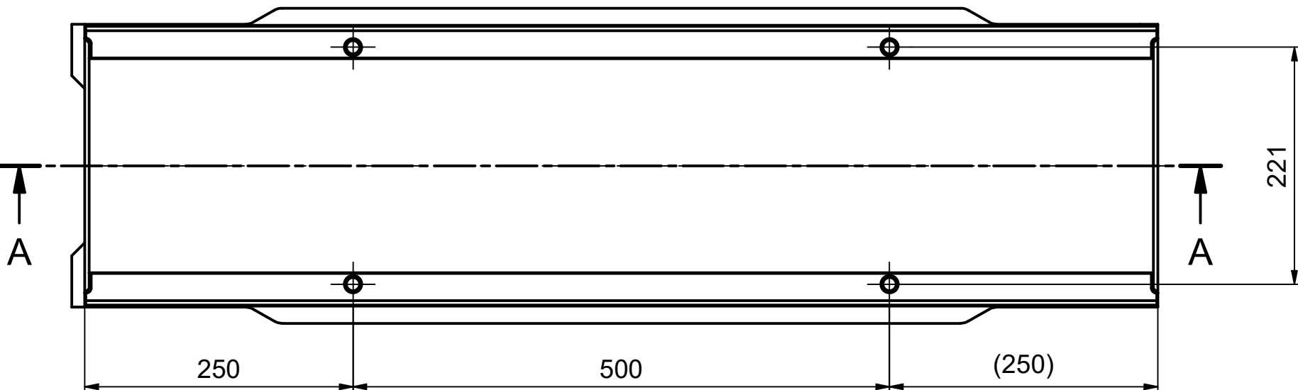
Draufsicht / top view / vue de dessus
