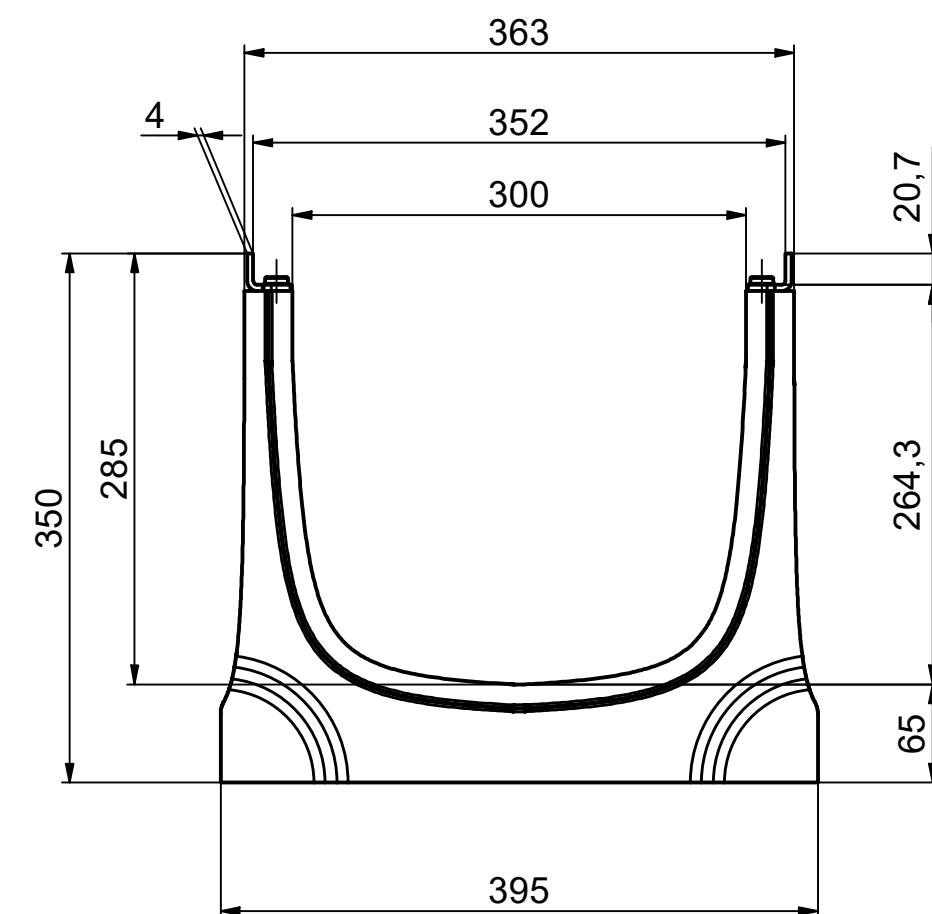
Ansicht Nut / view groove / vue rainure
