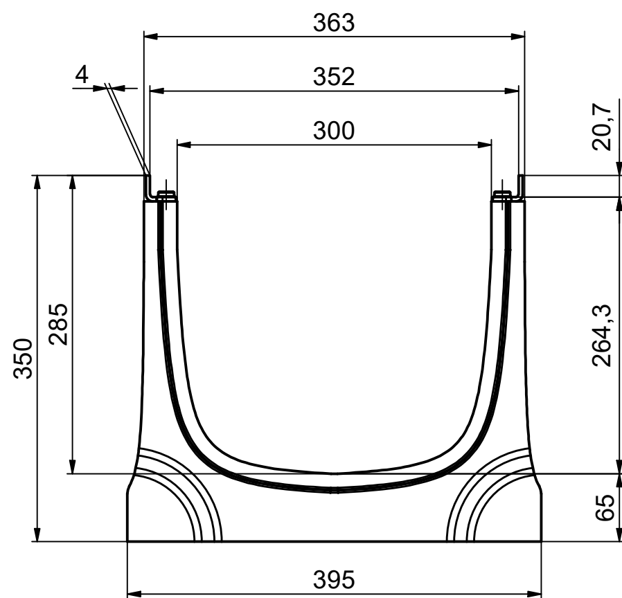
Ansicht Feder / view tongue / vue languette
