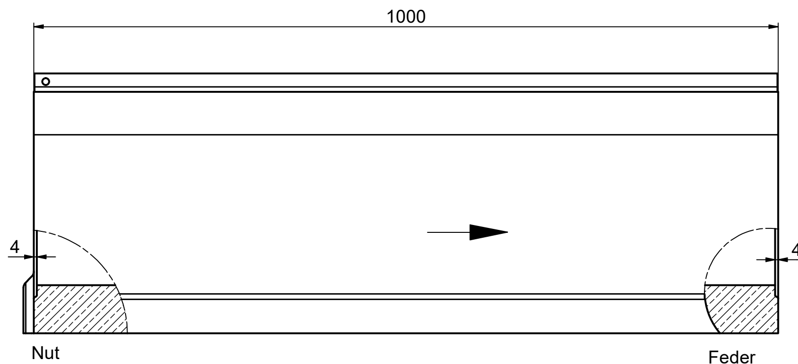
Seitenansicht / side view / vue de côté
