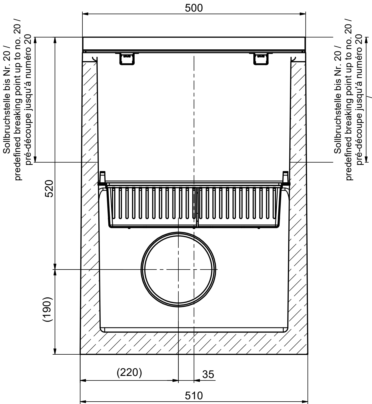
Schnitt / section / coupe B-B
