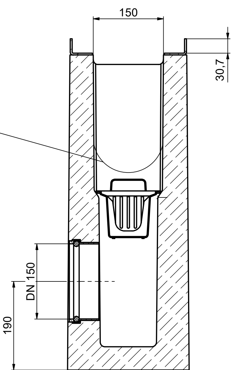
Schnitt / section / coupe C-C
