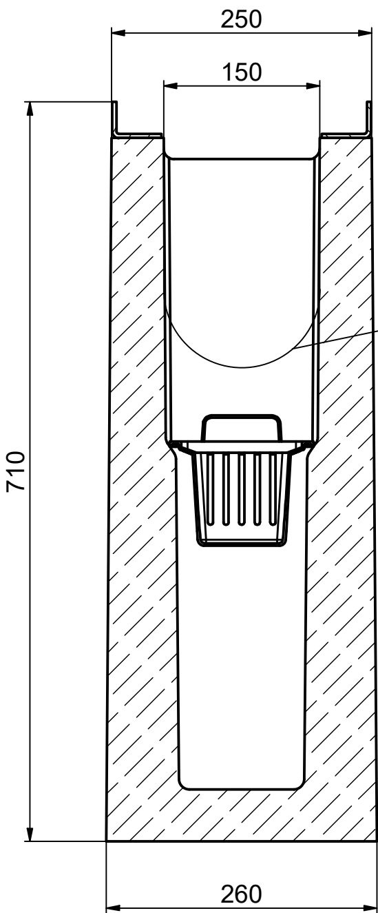
Schnitt / section / coupe A-A
